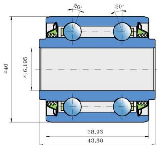
Rozměry/Dimensions (mm)
