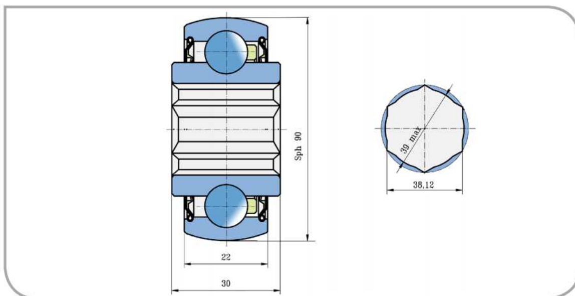
Rozměry/Dimensions (mm)
