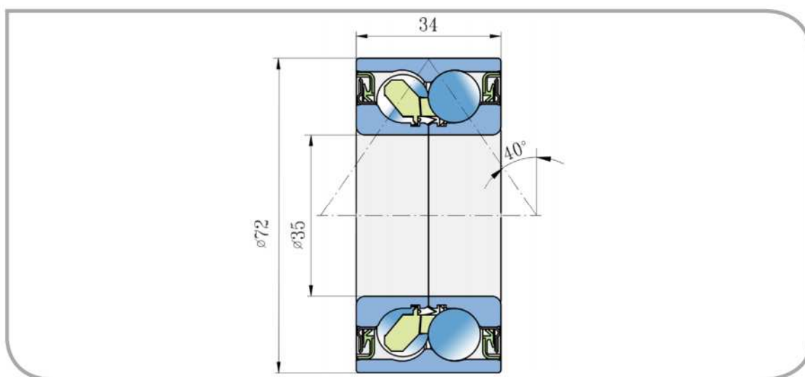
Rozměry/Dimensions (mm)
