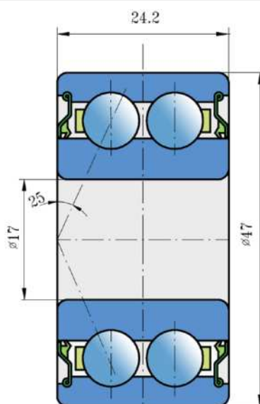
Rozměry/Dimensions (mm)
