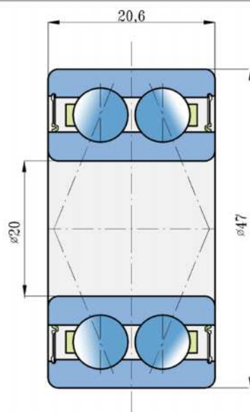
Rozměry/Dimensions (mm)
