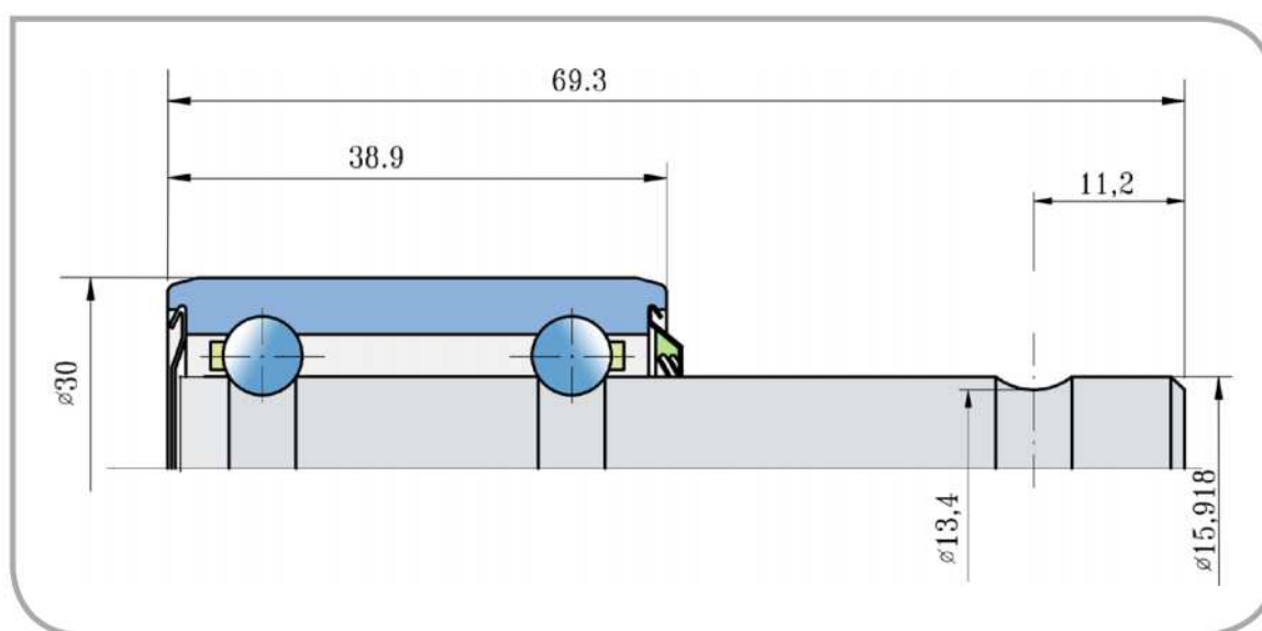
Rozměry/Dimensions (mm)
