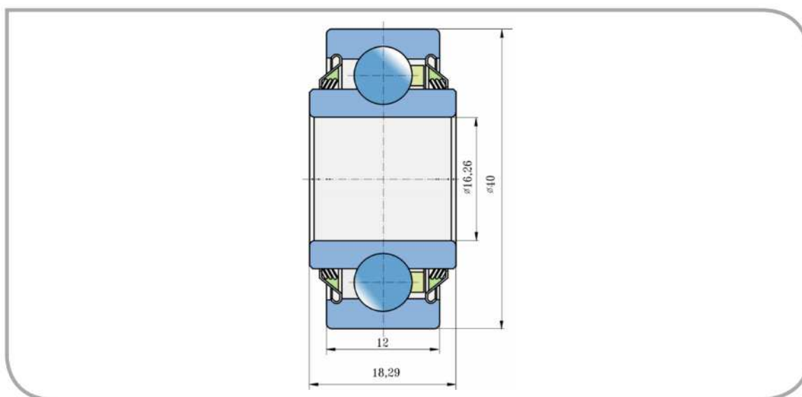
Rozměry/Dimensions (mm)
