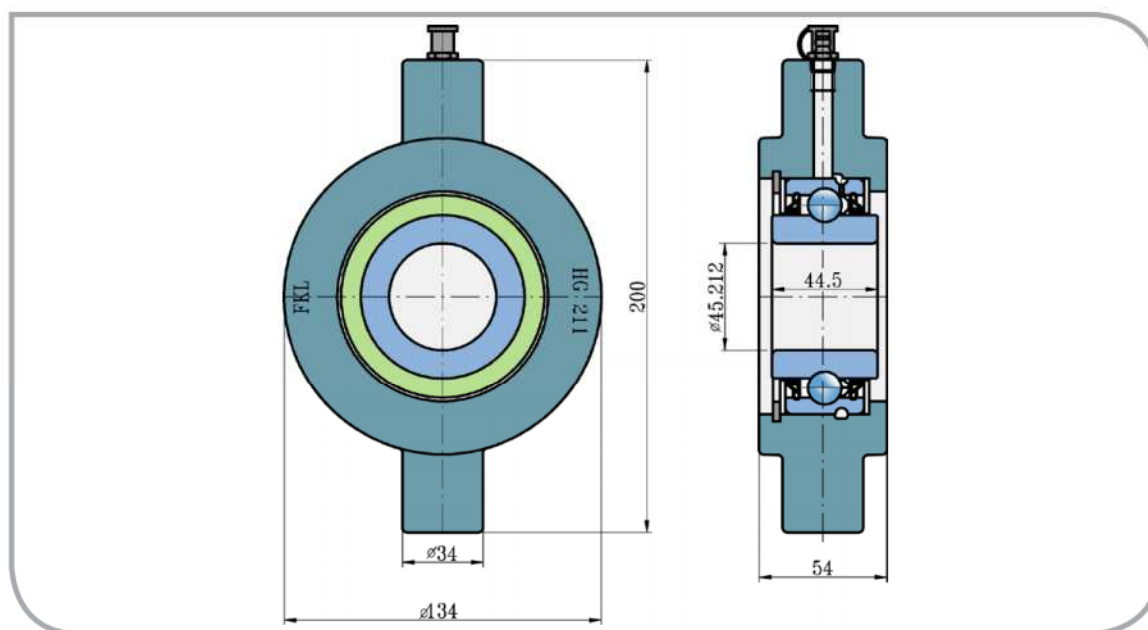
Rozměry/Dimensions (mm)
