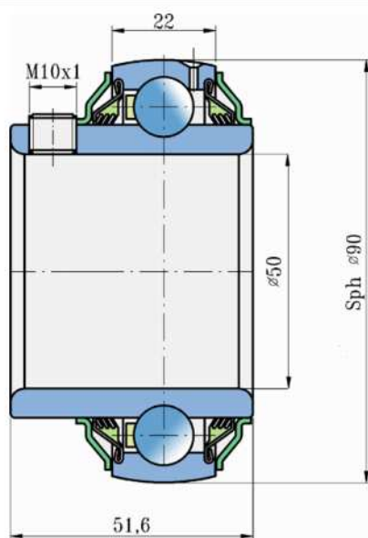
Rozměry/Dimensions (mm)
